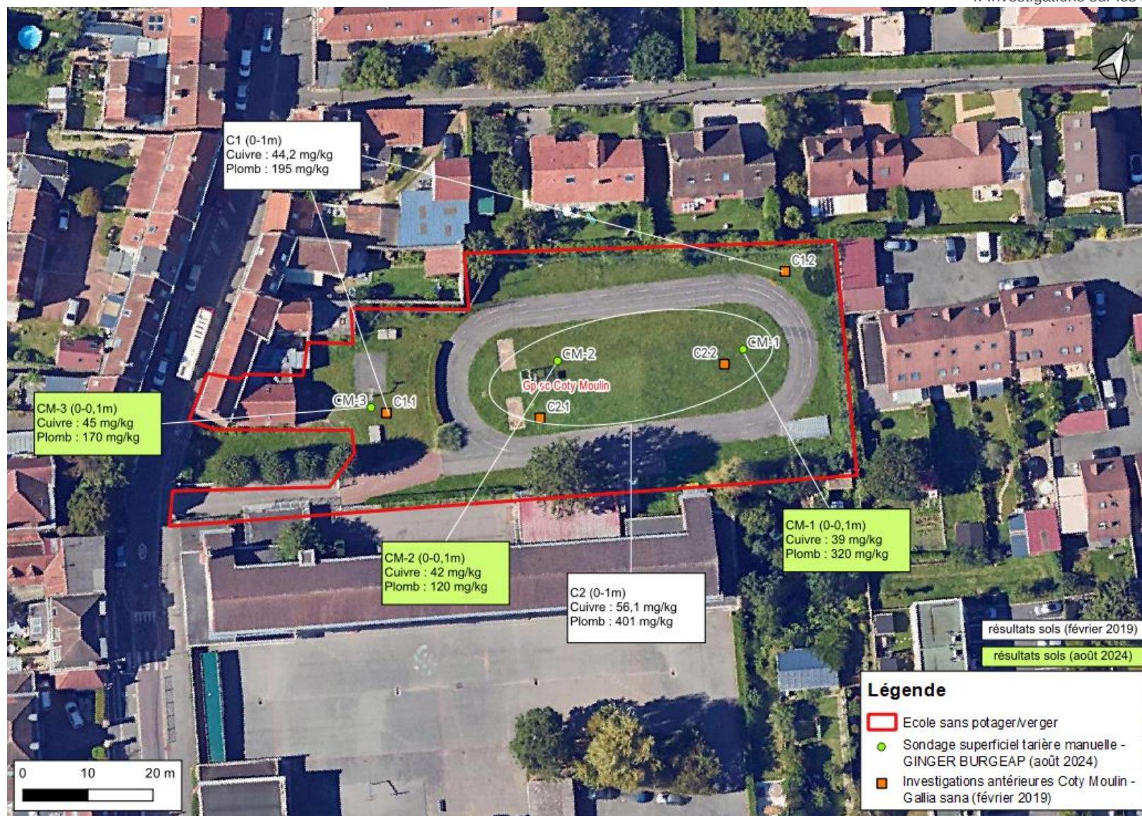
Figure 5 : Cartographie des anomalies dans les sols – Groupe scolaire Coty Moulin (GINGER BURGEAP, août 2024)
